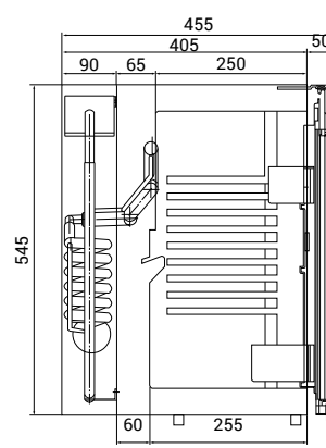
▼ bokorys TM 42
