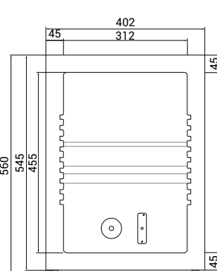
▼ bokorys TM 42
